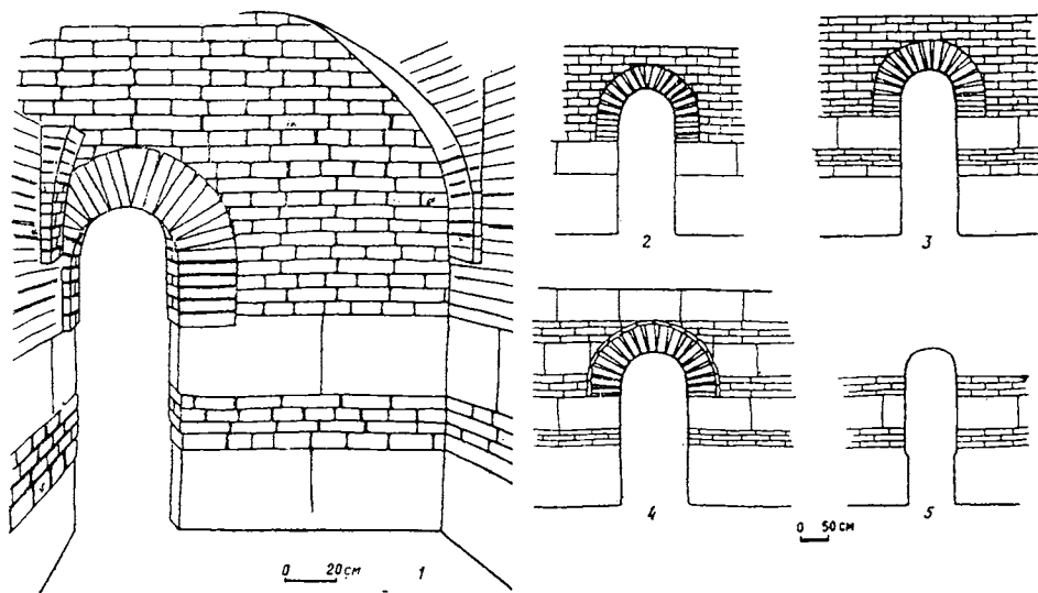
Рис. 30. Кладка стен и типы арочных проходов замка Луговое А. VII—VIII вв.
