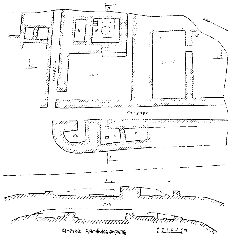
Рис. 19. План и разрезы конструкций нижнего строительного горизонта цитадели Куйрук-тобе. VII — первая половина IX в.
