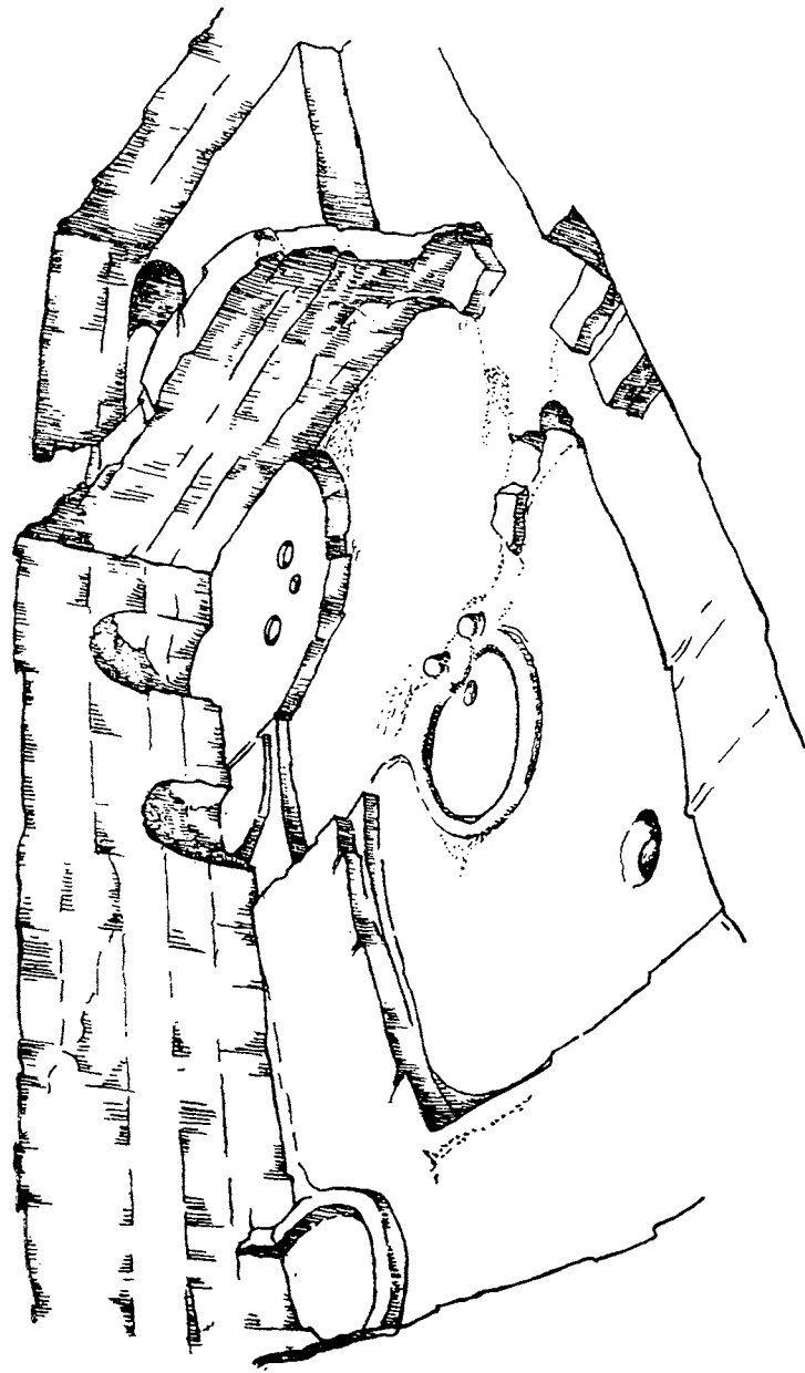
Рис. 87. Куйрук-тобе. Интерьер дома X — первой половины XI в.
